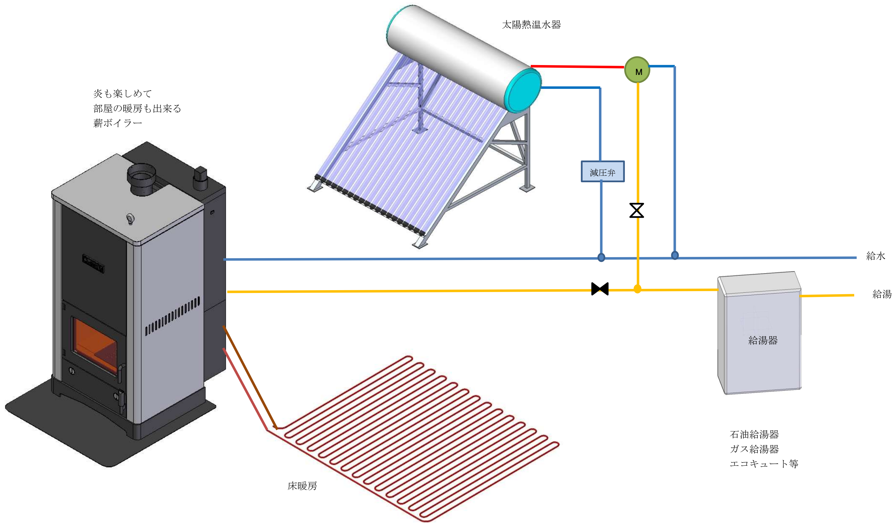
一般的な マキキュート配管図
