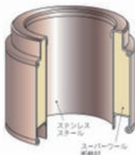
断熱二重管構造図
